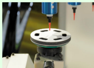
抛光液供应(注射器)
